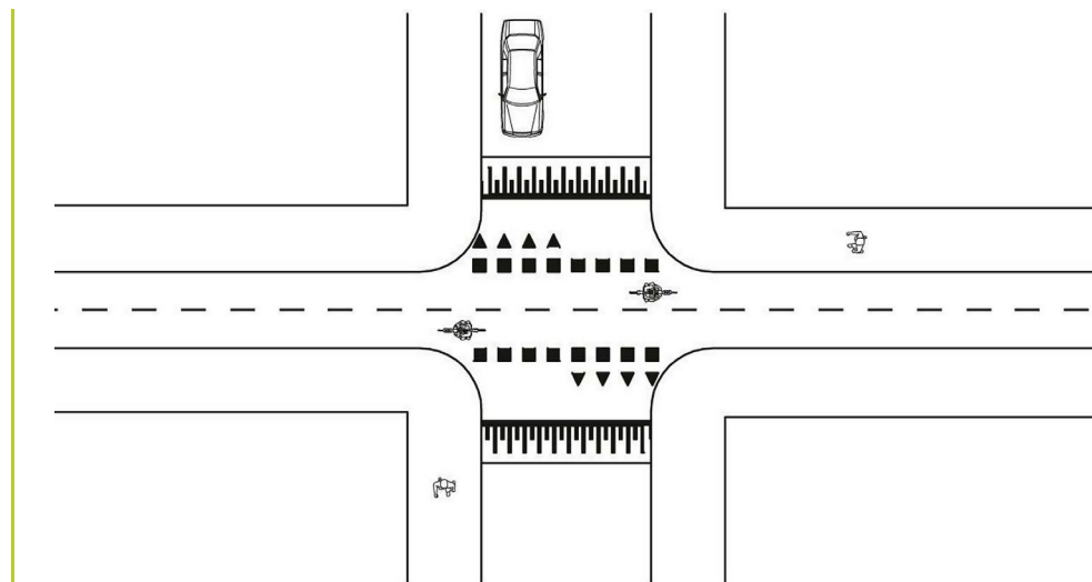
Afbeelding 4.1. Oversteek solitair fietspad met plateau volgens ASVV 14.2.15 (CROW, 2021)
