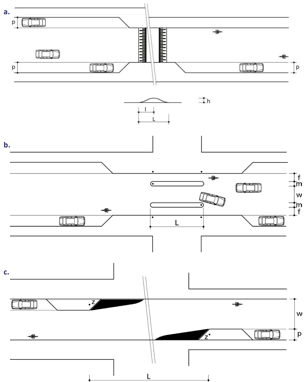
Afbeelding 4.3. Snelheidsremmers op erfgoedwegen binnen de bebouwde kom volgens ASVV 11.2.21, 11.2.24, 11.2.25 (CROW, 2021)
