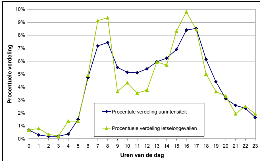
Afbeelding 5.3. Procentuele uurverdelingen van de intensiteiten en het aantal letselongevallen gemiddeld voor werkdagen in de periode 1997 tot en met 2003 op de meetvakken van de provinciale enkelbaanswegen in Noord-Holland.
