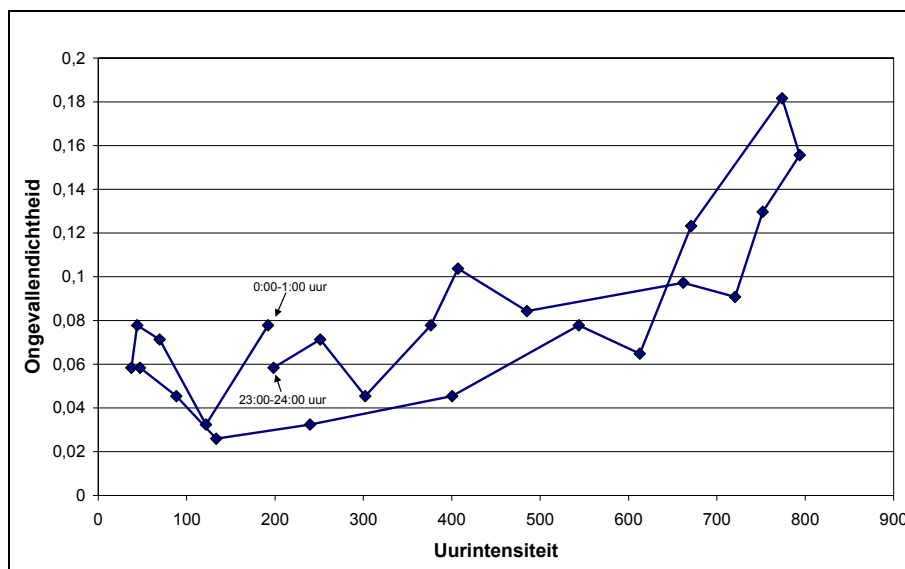
Afbeelding 5.10. De ongevallendichtheden voor de uren van de weekenddag uitgezet tegen de uurintensiteit, gemiddeld voor de jaren 1997 tot en met 2003 van de meetvakken op de provinciale enkelbaanswegen in Noord-Holland.
