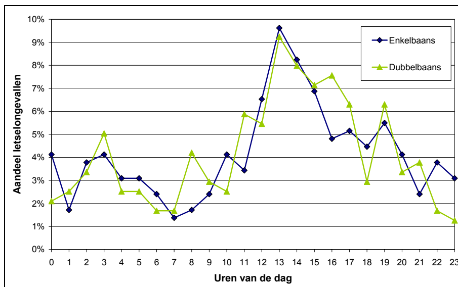
Afbeelding 4.8. Procentuele uurverdelingen van de letselongevallen op weekenddagen, gemiddeld voor de periode 1997 tot en met 2003 op de meetvakken van provinciale wegen in Noord-Holland.
