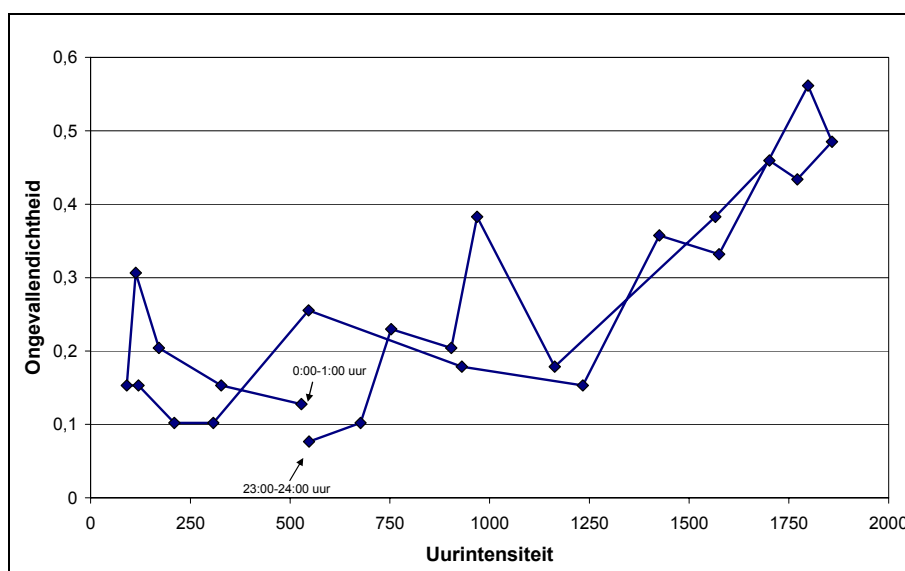
Afbeelding 5.11. De ongevallendichtheden voor de uren van de weekenddag uitgezet tegen de uurintensiteit, gemiddeld voor de jaren 1997 tot en met 2003 van de meetvakken op de provinciale dubbelbaanswegen in Noord-Holland.
