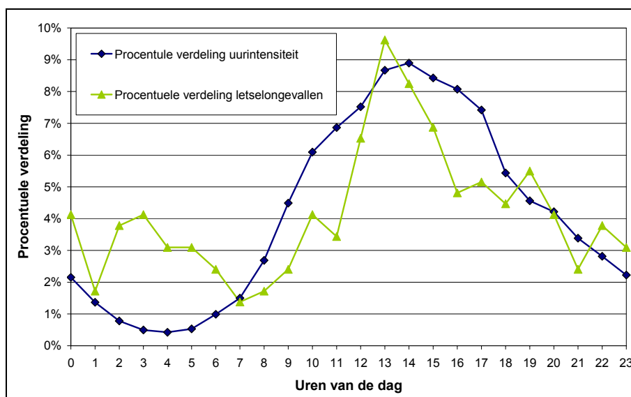
Afbeelding 5.5. Procentuele uurverdelingen van de intensiteiten en het aantal letselongevallen gemiddeld voor weekenddagen in de periode 1997 tot en met 2003 op de meetvakken van de provinciale enkelbaanswegen in Noord-Holland.
